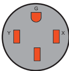
NEMA L14-50
